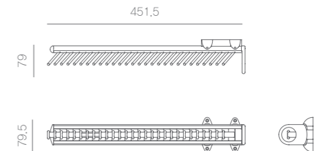
Slim Tie Hanger / D1-GITG-SM
