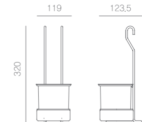
1-Cup Spoon Container / D2-AST-S
