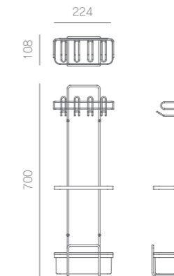
B TYPE D1-UEW-B
